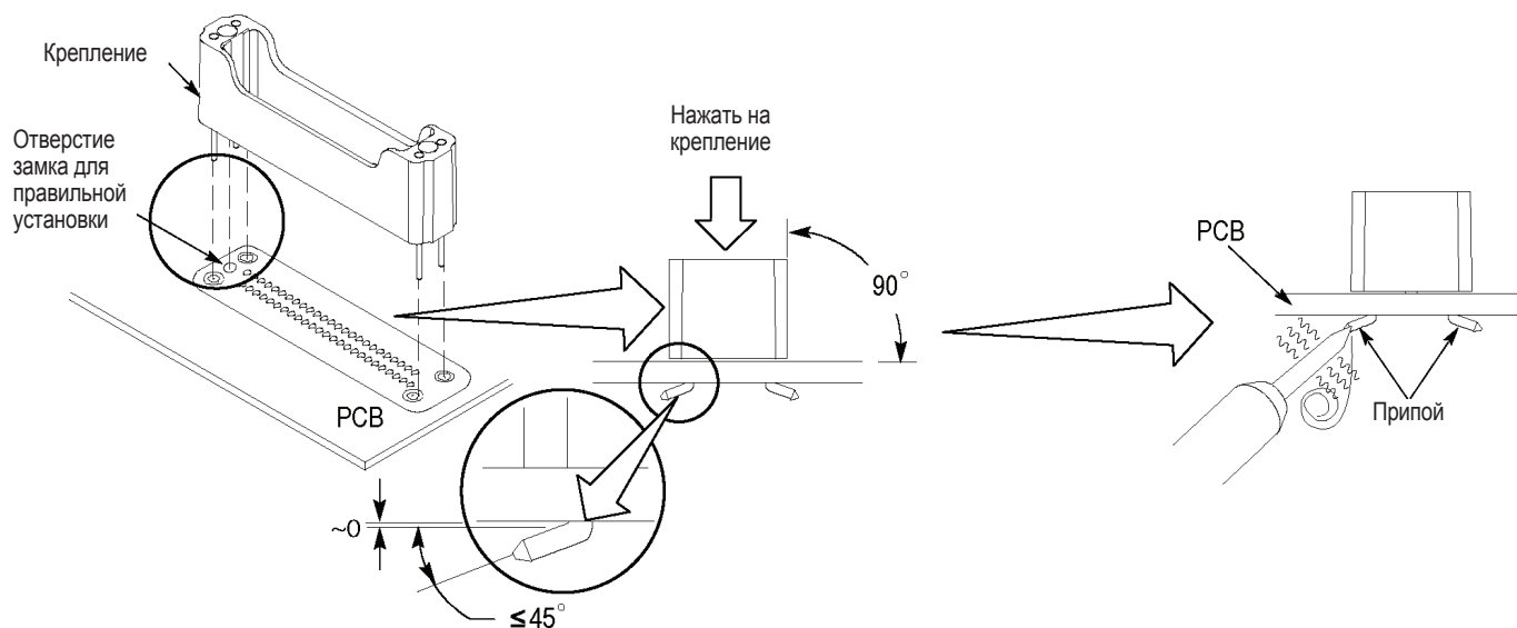
Крепление для пробника P69xx
